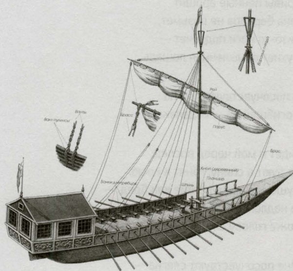
Схема струга
