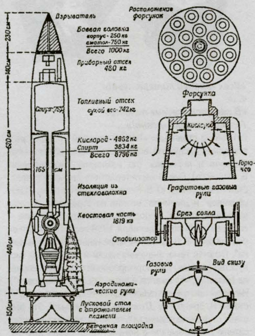
Схема баллистической ракеты «Фау-2»
